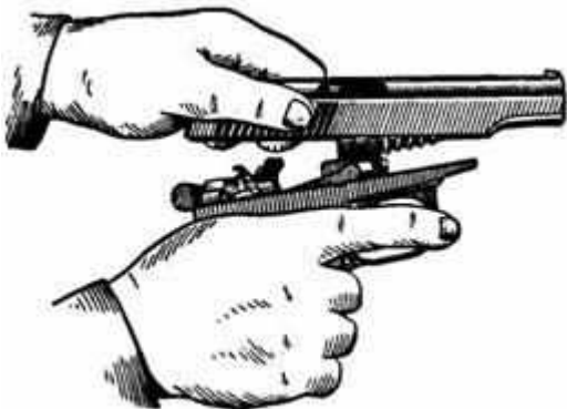
Рис. Введение свободного конца возвратной пружины в канал затвора
