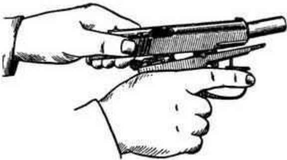
Рис. Отделение затвора от рамки
