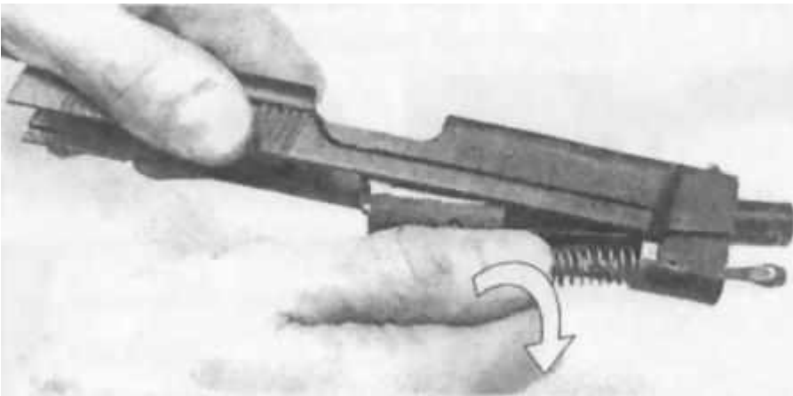
Рис. Отсоединение ствола со штоком и возвратной пружиной от затвора
