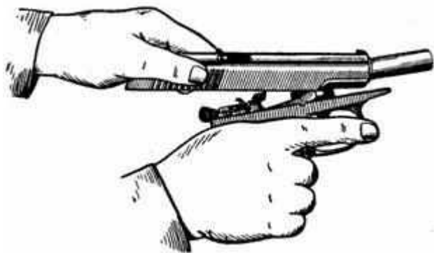
Рис. Присоединение затвора к рамке
