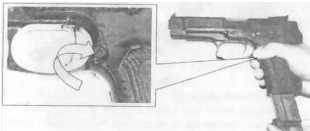
Рис.1 Отсоединение магазина
